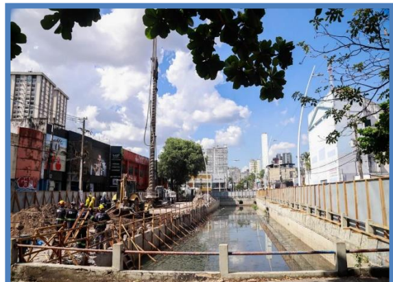
FOTO 38: Serviços de fundação: perfuração de estacas hélices.
