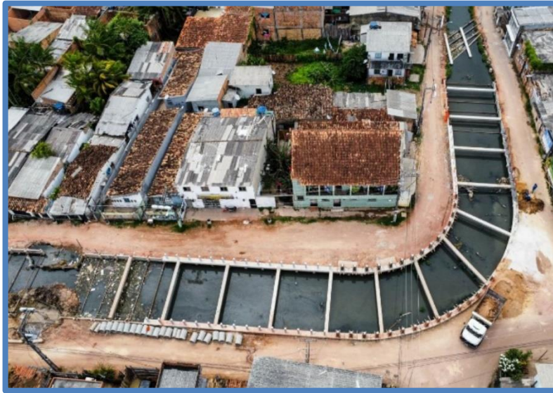
FOTO 57: Execução das fundações das pontes e passarelas, cravação de estacas de concreto, placas e vigas de coroamento.
