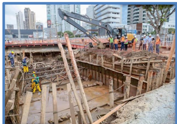
FOTO 36: Serviços de fundação, lançamento e concretagem das peças metálicas, e cravação de estacas de sustentação da estrutura do canal.
